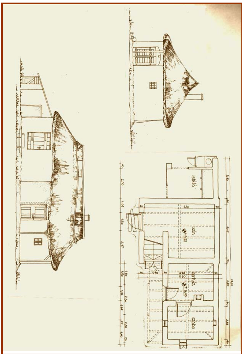
Tóth Sandorné báromsejtű, nádfedezés, tornácos, pincés pajtájának alaprajza és homlokzatai
